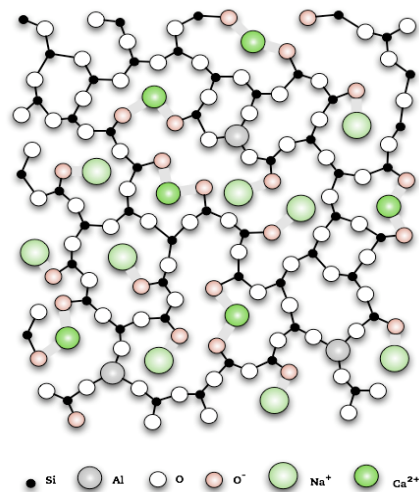
ソーダ石灰ガラス
