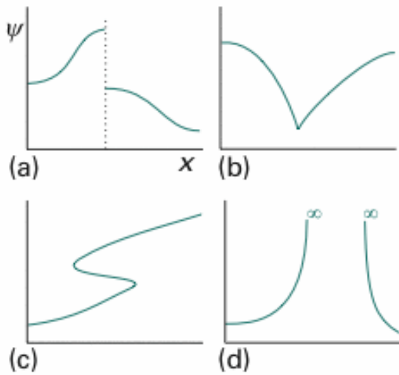
図2. 波動関数として許されない関数の例
