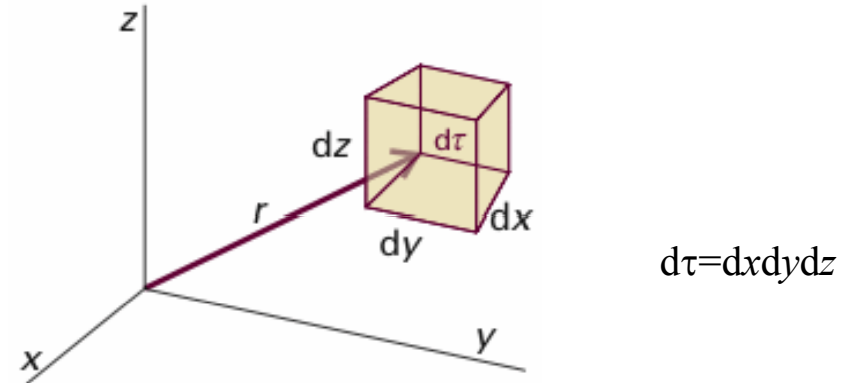
8・20 3次元空間における波動関数のボルンの解釈。
