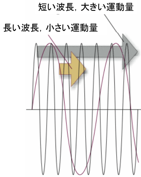
図8・16 運動量と波長の間 ドブローイの関係式を示した図。 波が粒子に伴う(この波は、粒 子の波動関数であることがすぐ にわかる)。大きい運動量をも つ粒子は波長の短い波動関数 をもっている。その逆も正しい。
