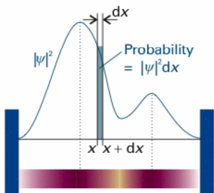
図8・19 波動関数 \psi は、その絶対値の自乗 \psi^* \psi または |\psi|^2 が確率密度であるという意味で確率振幅である。位置xにおける領域dxに粒子を見出す確率は |\psi|^2 dx に比例する。
