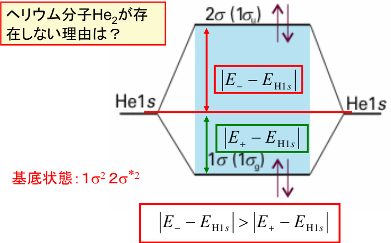
図11・24 Heの1sオービタルの重なりから作られたヘリウム分子の分子オービタルのエネルギー準位図. ヘリウム分子のエネルギーは2つの孤立したヘリウム原子のエネルギーの和より高く不安定なのでヘリウム分子を形成しない.
