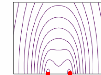
図11・13 (a)水素分子イオンの2個の原子核を含む平面内における結合分子オービタル \psi_{+}
