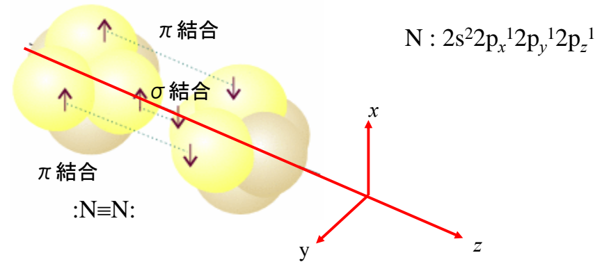
図11・5 窒素分子における結合の構造。σ結合1個とπ結合2個がある。総合的な電子密度は、結合軸の回りに円筒対称を持っている。同一線上にある2つのpオービタルの電子の間のオービタルの重なりとスピン対形成によって、σ結合が形成される。
