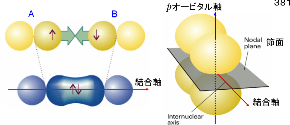
図11・4 結合軸に垂直な軸を持つpオービタルにある電子の間のオービタルの重なりとスピン対形成によって \pi 結合 ができる。
