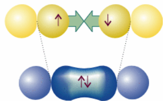
σ分子オービタル
