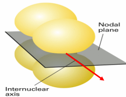
π分子オービタル
