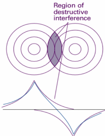
図11・18 2個のH1sオービタルが重なり合っ \sigma^* オービタル \psi_- を形成するとき弱め合う干渉が起こる。
