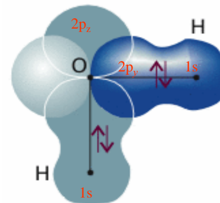
図11・6 原子価結合法によるH 2 O分子の結合の様子を表したもの。おのこのσ結合は、H1sオービタルとO2pオービタルの1個が重なることによってできる。
