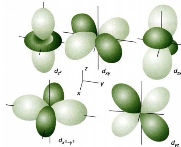
図10・16 dオービタルの境界面。2つの節面が原子核の位置で交差し、ローブを分断する。暗い部分と明るい部分は波動関数の符号が互いに反対であることを示している。
